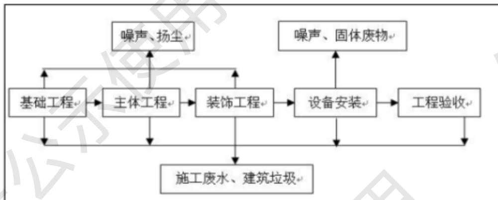
图 2.3.1-1 施工工艺流程图
