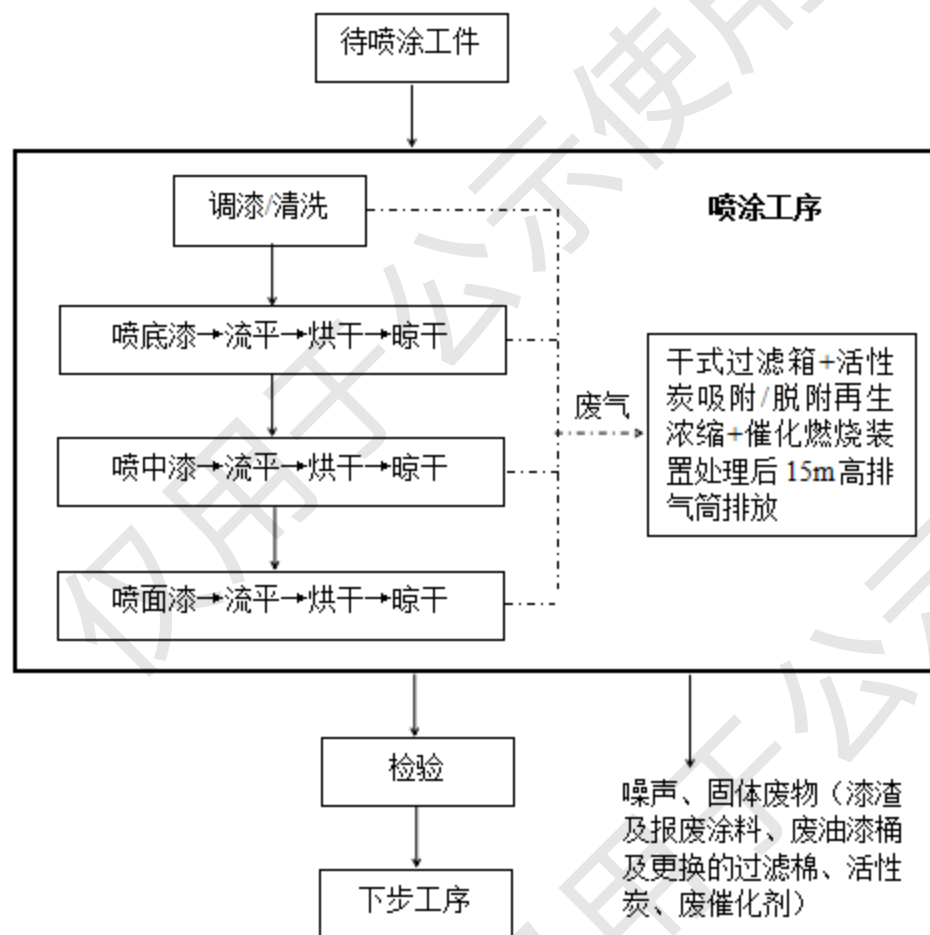
图 2.3.2-3 喷涂工艺流程图
